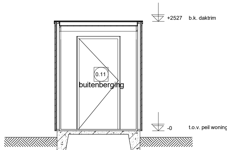
Doorsnede D1.1
