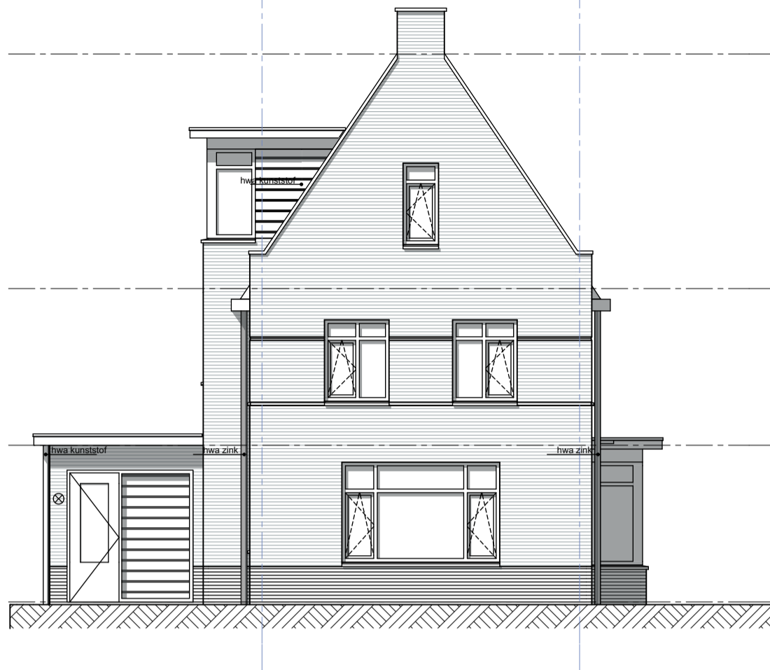
Vorgevel
