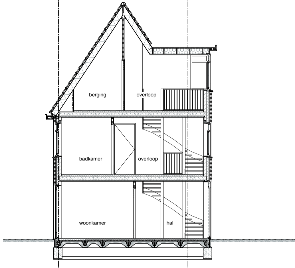
Doorsnede
