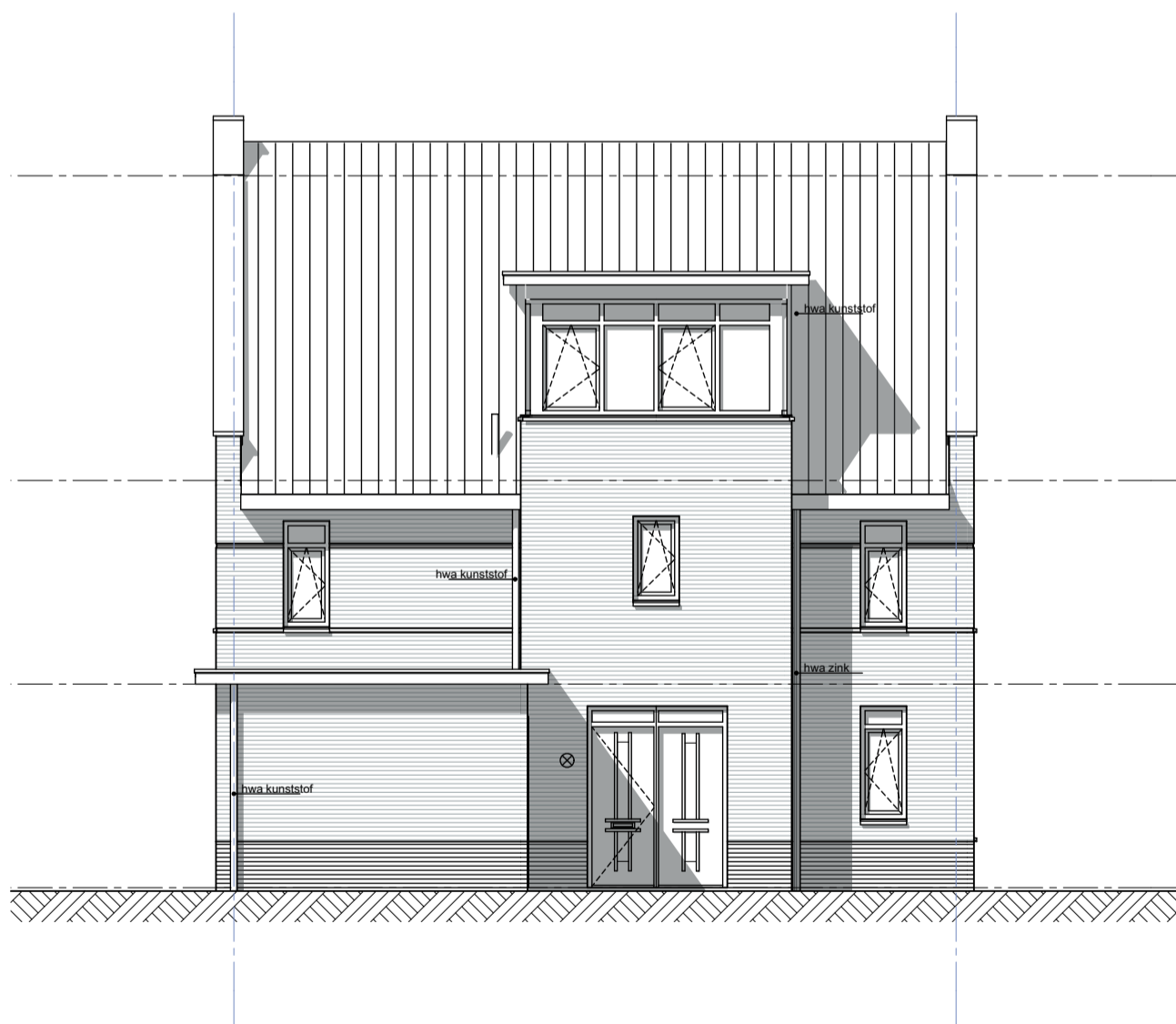
Linkergevel
