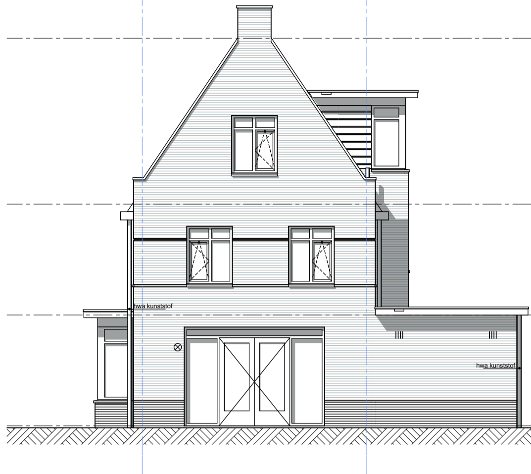
Achtergevel
