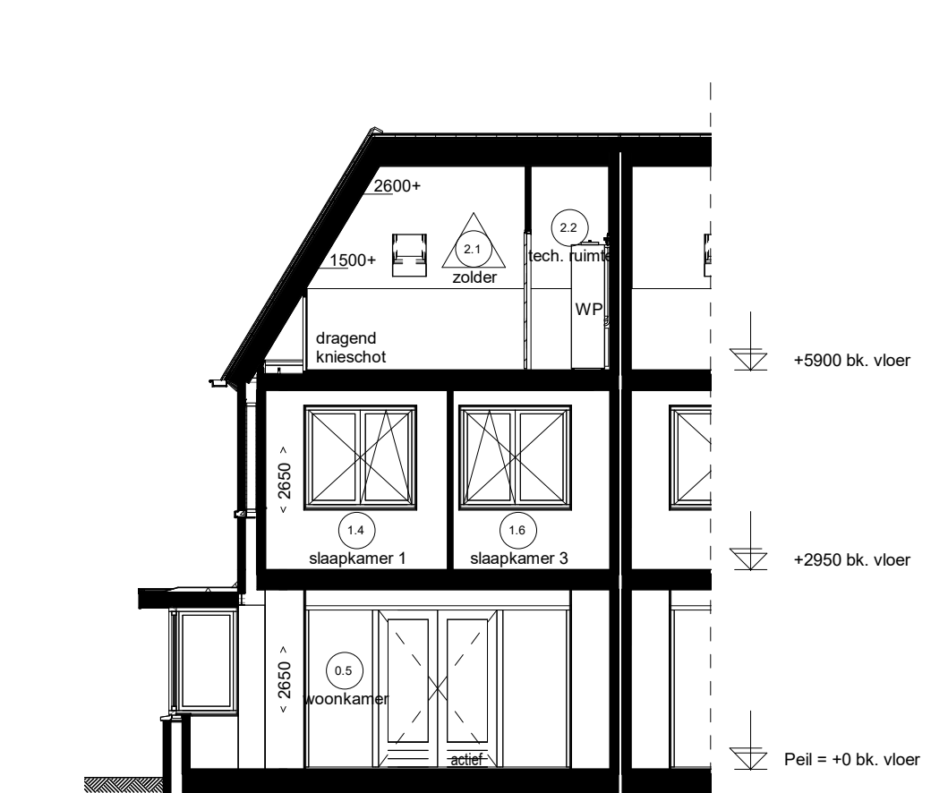
Doorsnede D1.D
