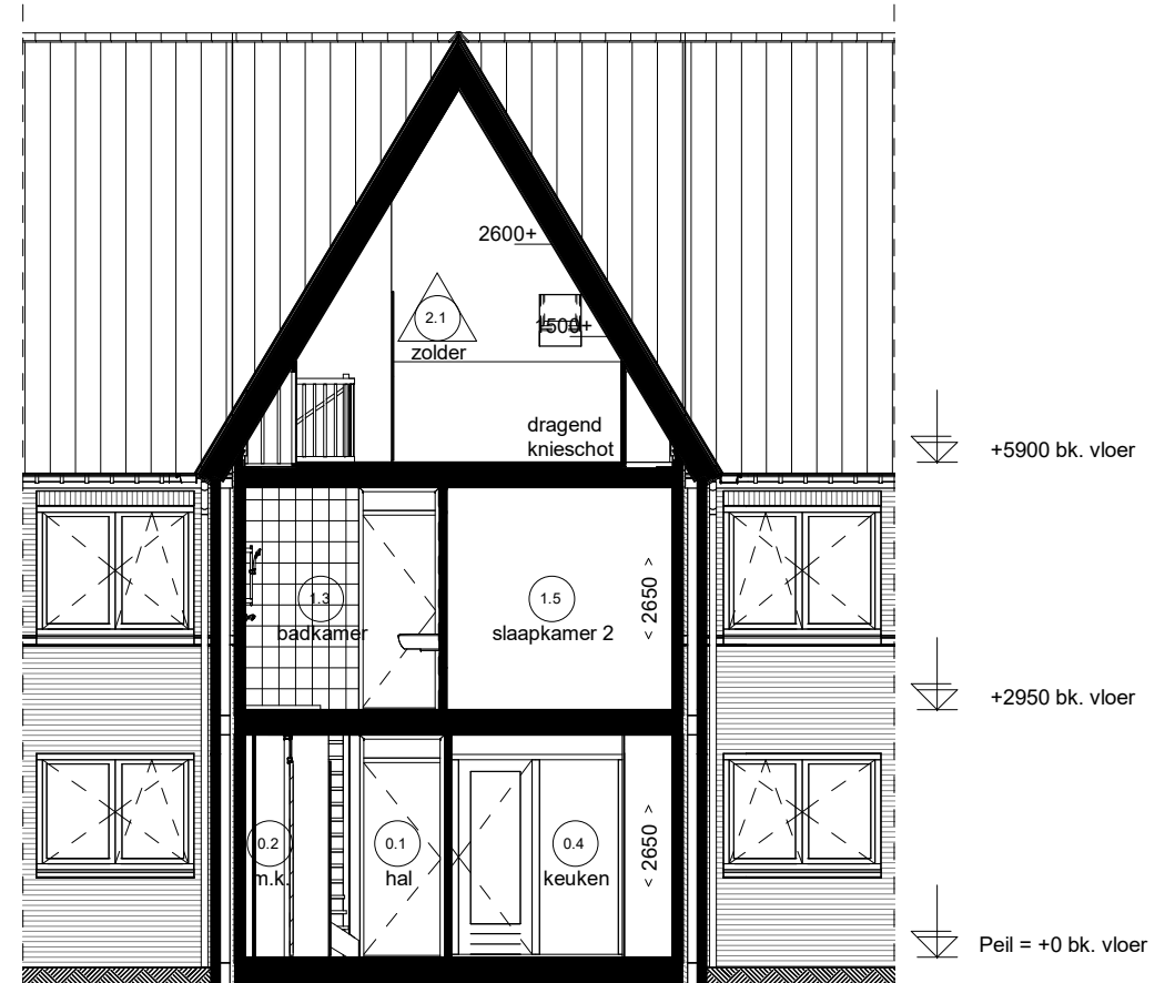
Doorsnede D1.C
