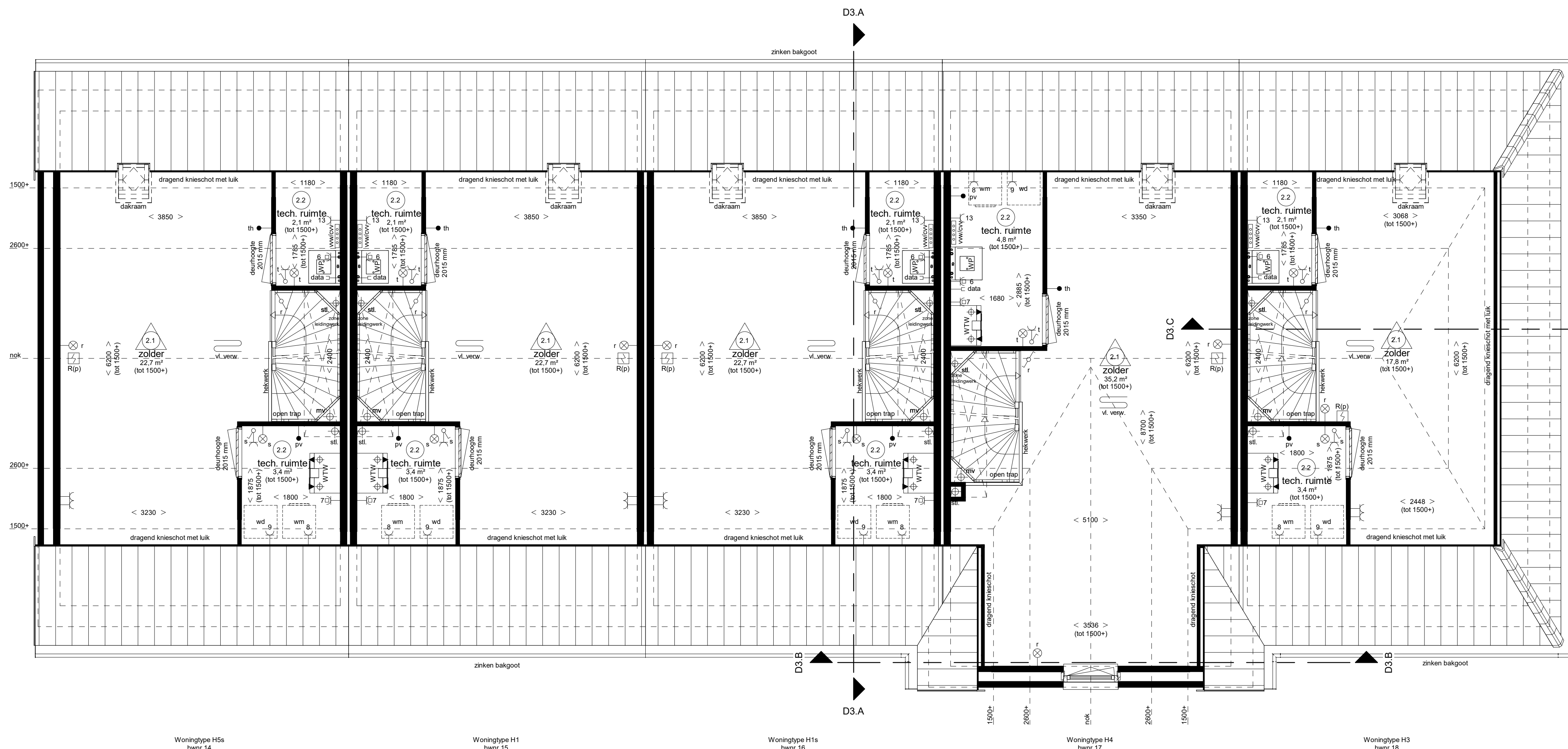
Tweede verdieping
