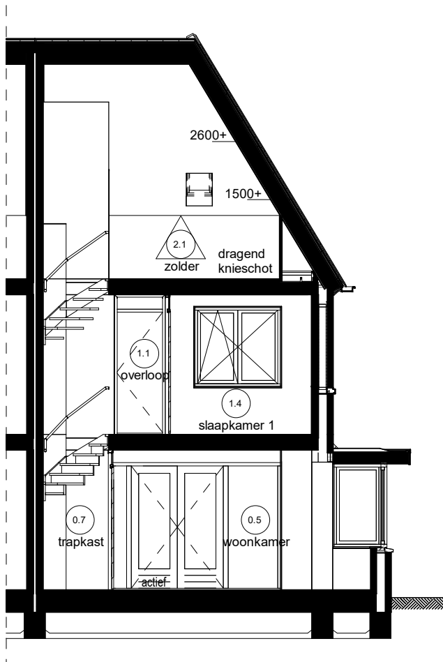
Doorsnede D5.C
