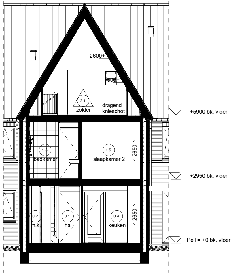
Doorsnede D5.B
