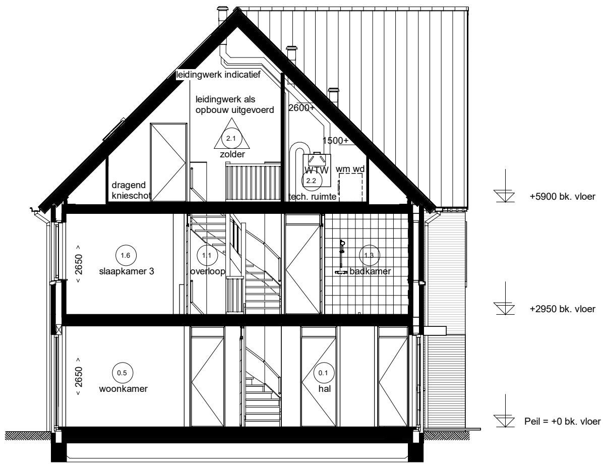
Doorsnede D5.A
