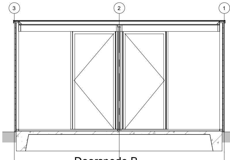
Doorsnede B
