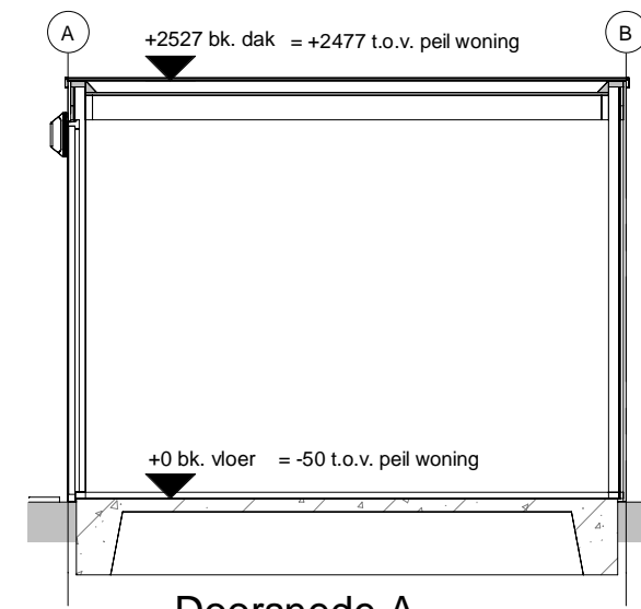
Doorsnede A
