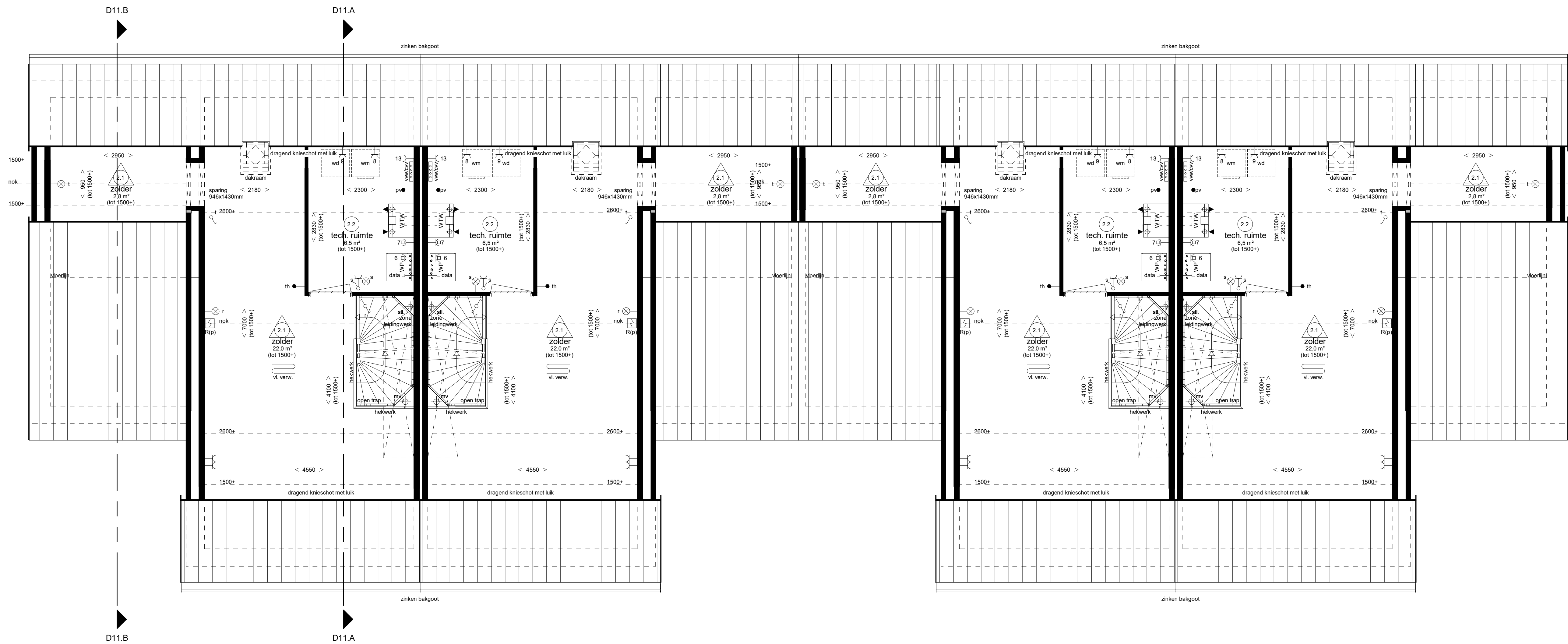
Tweede verdieping
