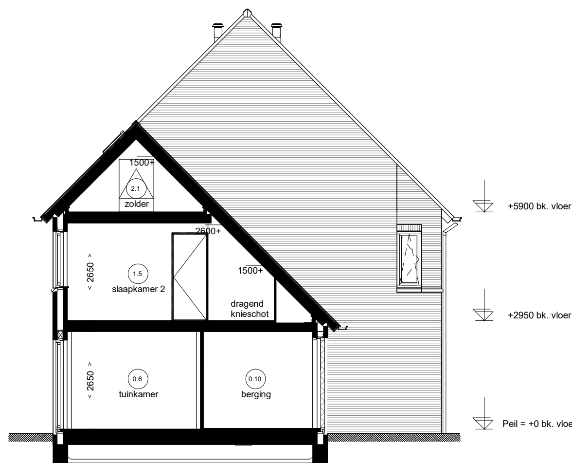
Doorsnede D11.B
