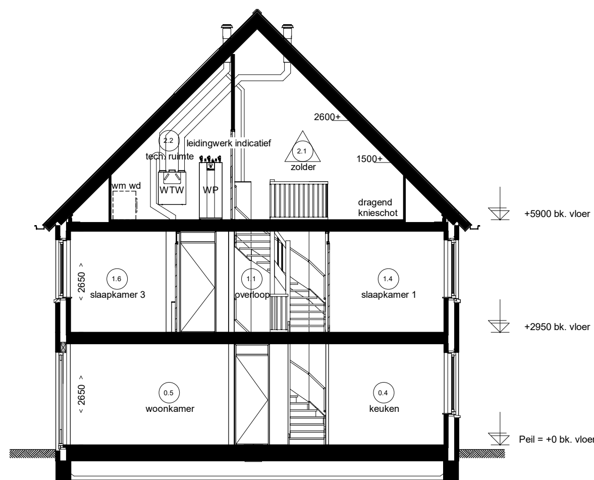
Doorsnede D11.A
