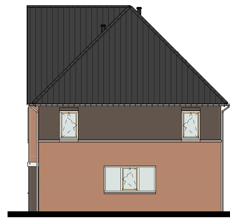
Rechtergevel
