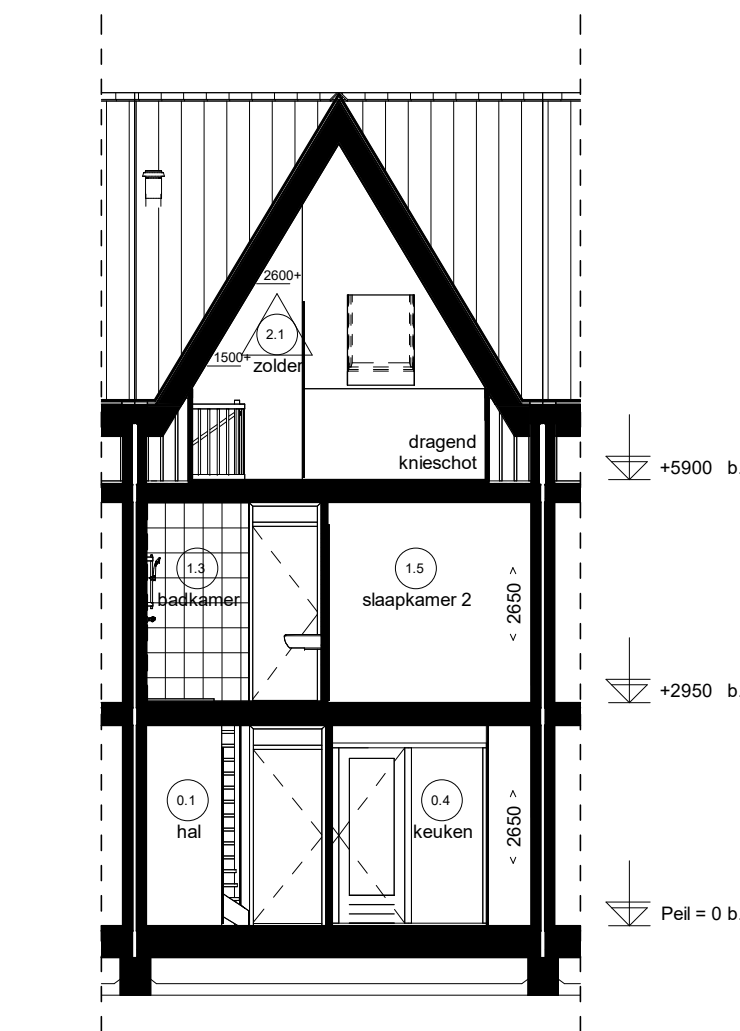
Doorsnede D05.D
