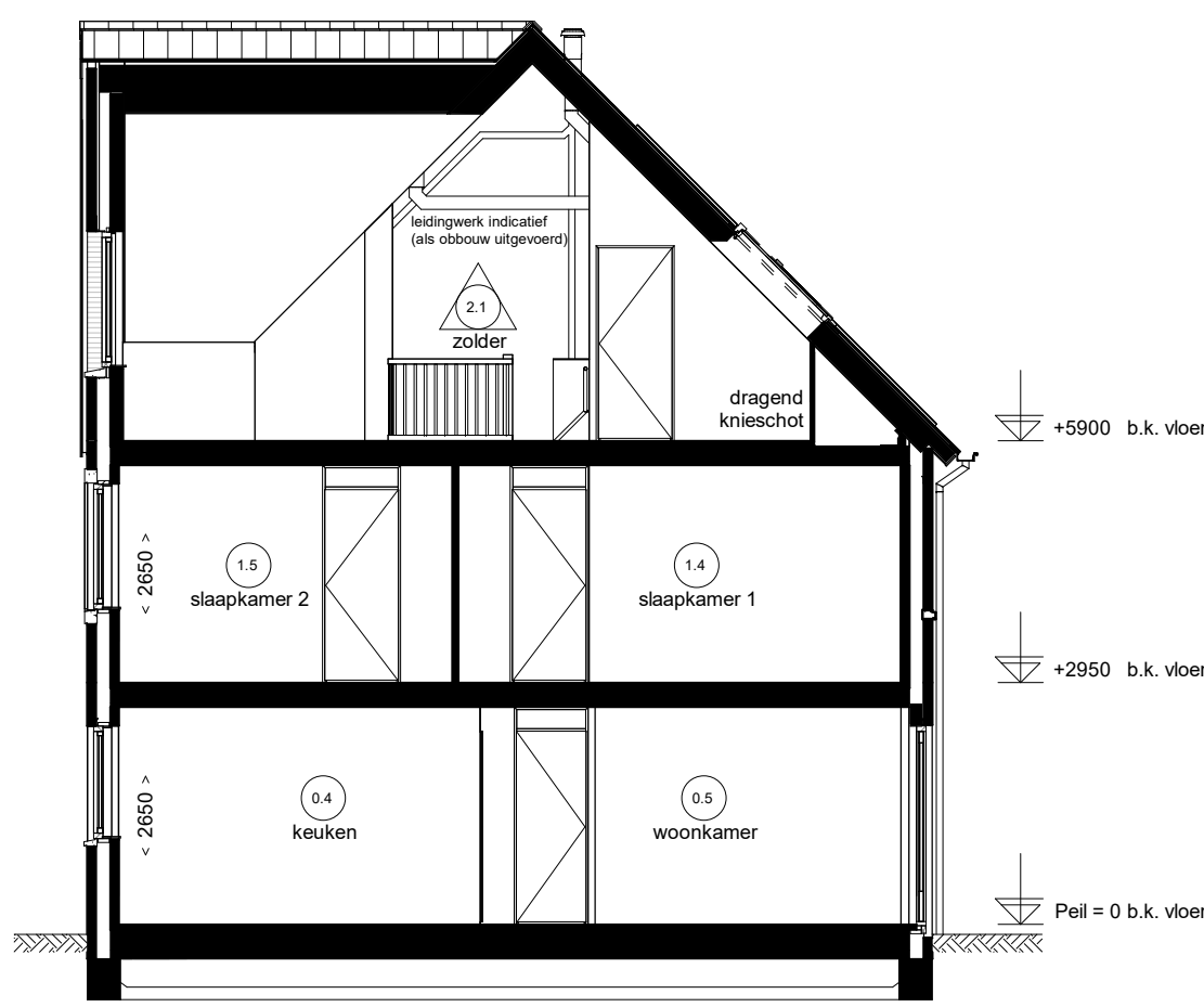
Doorsnede D05.B
