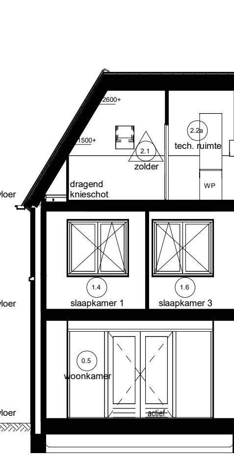
Doorsnede D05.C
