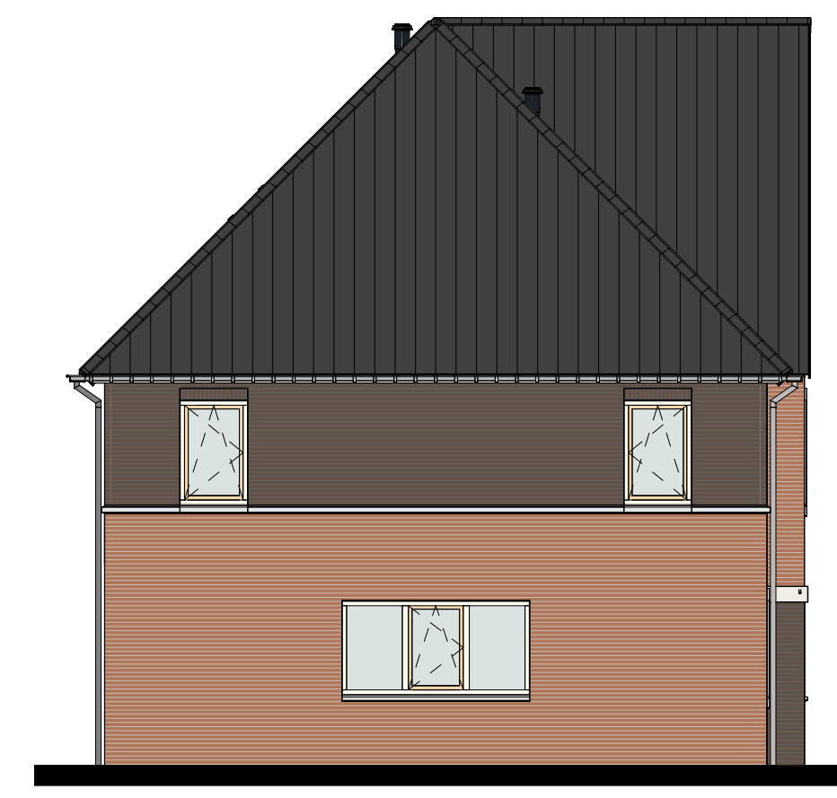
Linkergevel
