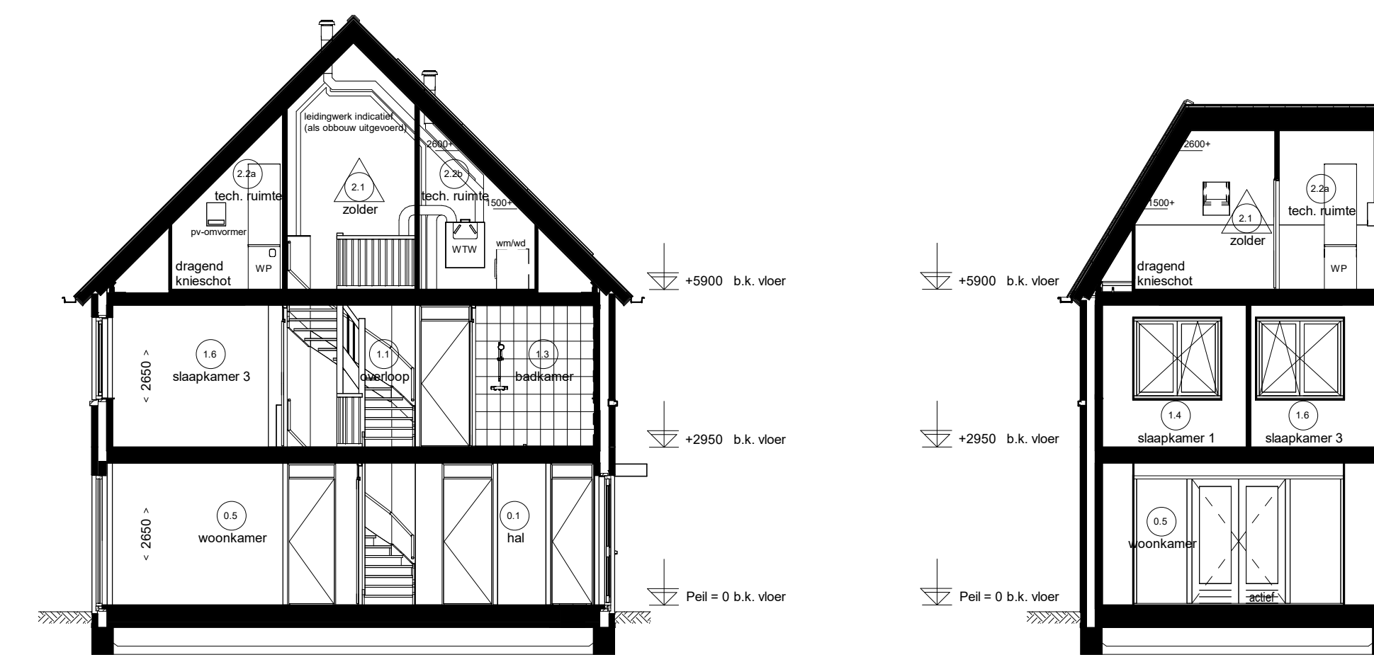
Doorsnede D05.A
