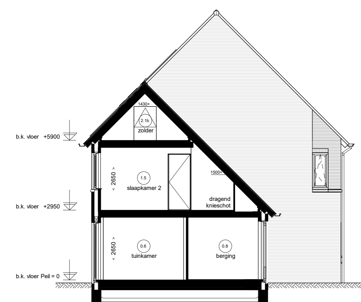
Doorsnede D01.A
