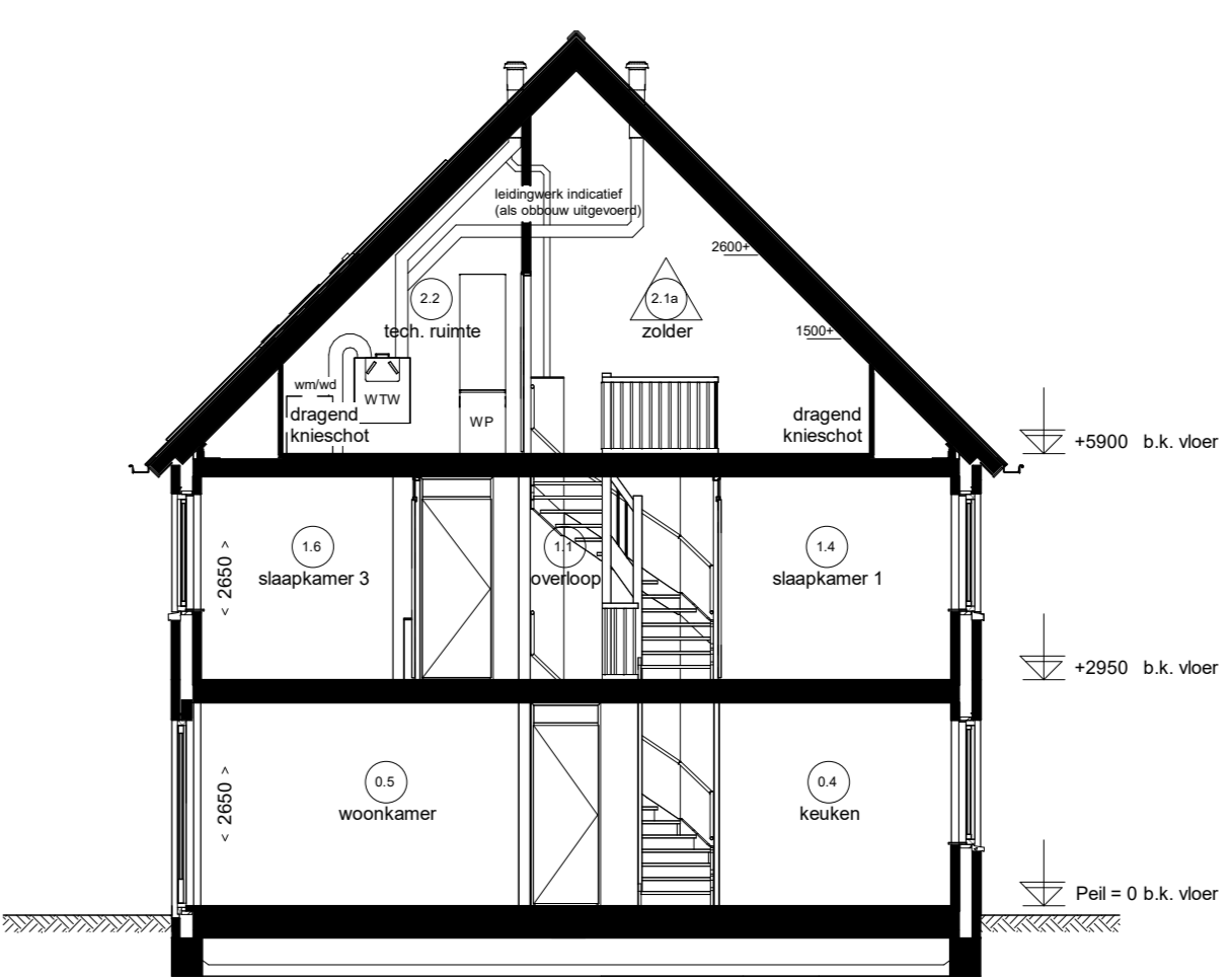
Doorsnede D01.B
