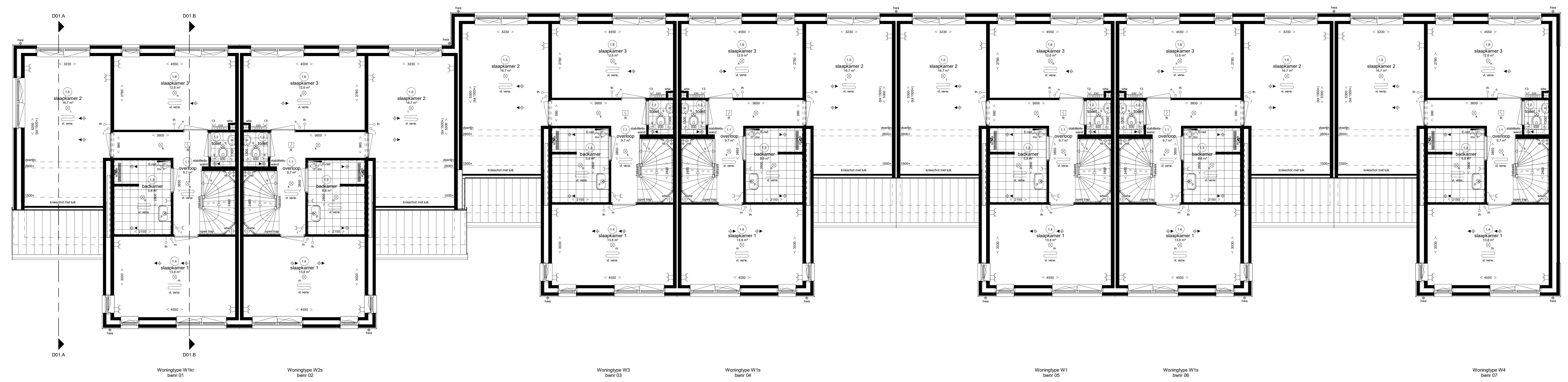
Eerste verdieping
