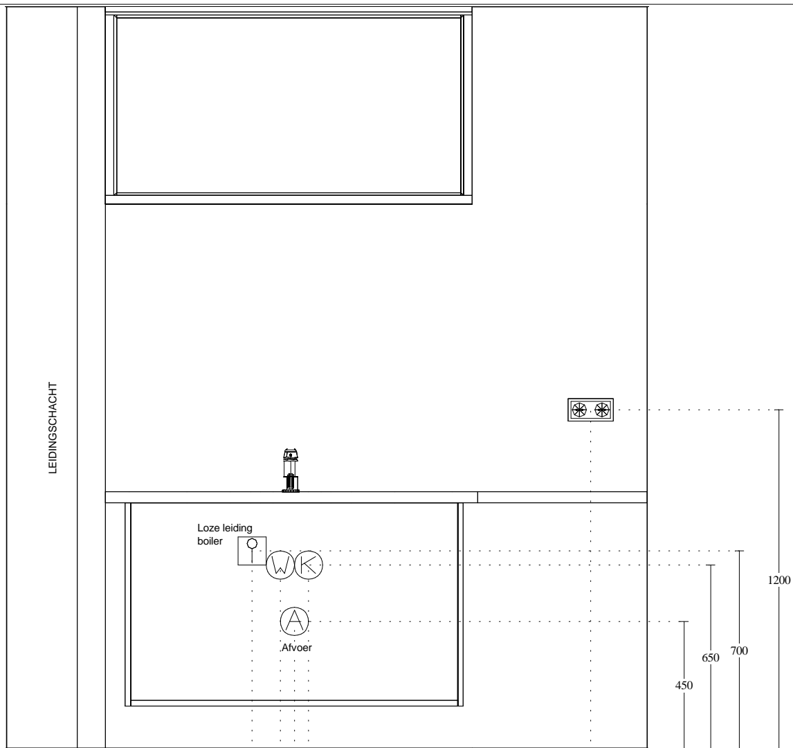
WANDAANZICHT A
